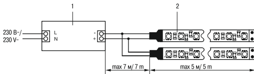
Рисунок 1 – Схема подключения одноцветной светодиодной ленты / Figure 1 – Connection diagram of monochrome LED strip / 1-sýret – Birtústi jaryqdiody taspany qosý sulbasy / Рисунок 1 – Схема підключення одноколірної світлодіодної стрічки
