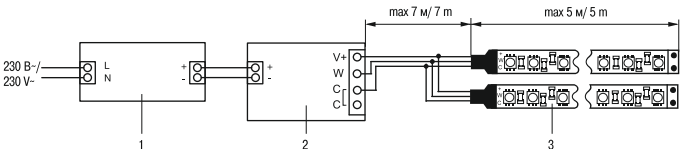
Рисунок 2 – Схема подключения RGB светодиодной ленты к блоку питания и контроллеру / Figure 2 – Connection diagram of RGB LED strip to the power supply unit and controller / 2-sýret – RGB jaryqdiody taspany qyat berý blogy men baqýlaýyshqa qosý sulbasy / Рисунок 2 – Схема підключення RGB світлодіодної стрічки до блоку живлення та контролера
