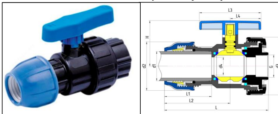
Рисунок 6. Кран шаровой цапга-внутренняя резьба
