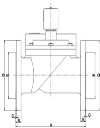
Рисунок 1. Эскиз
