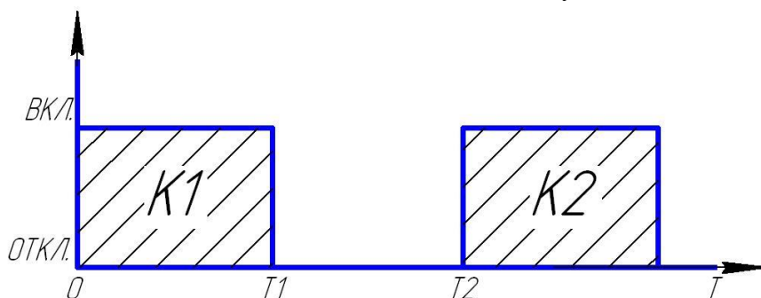
Рис.1. Диаграмма переключения выходных реле РТ-015.
