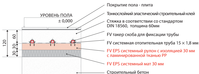
Рисунок 17: Рекомендуемый состав пола в подвальных и малоотпливаемых помещениях в соответствии со стандартом ČSN EN 1264 термостойкость изоляции R=1,25 м² К/В
