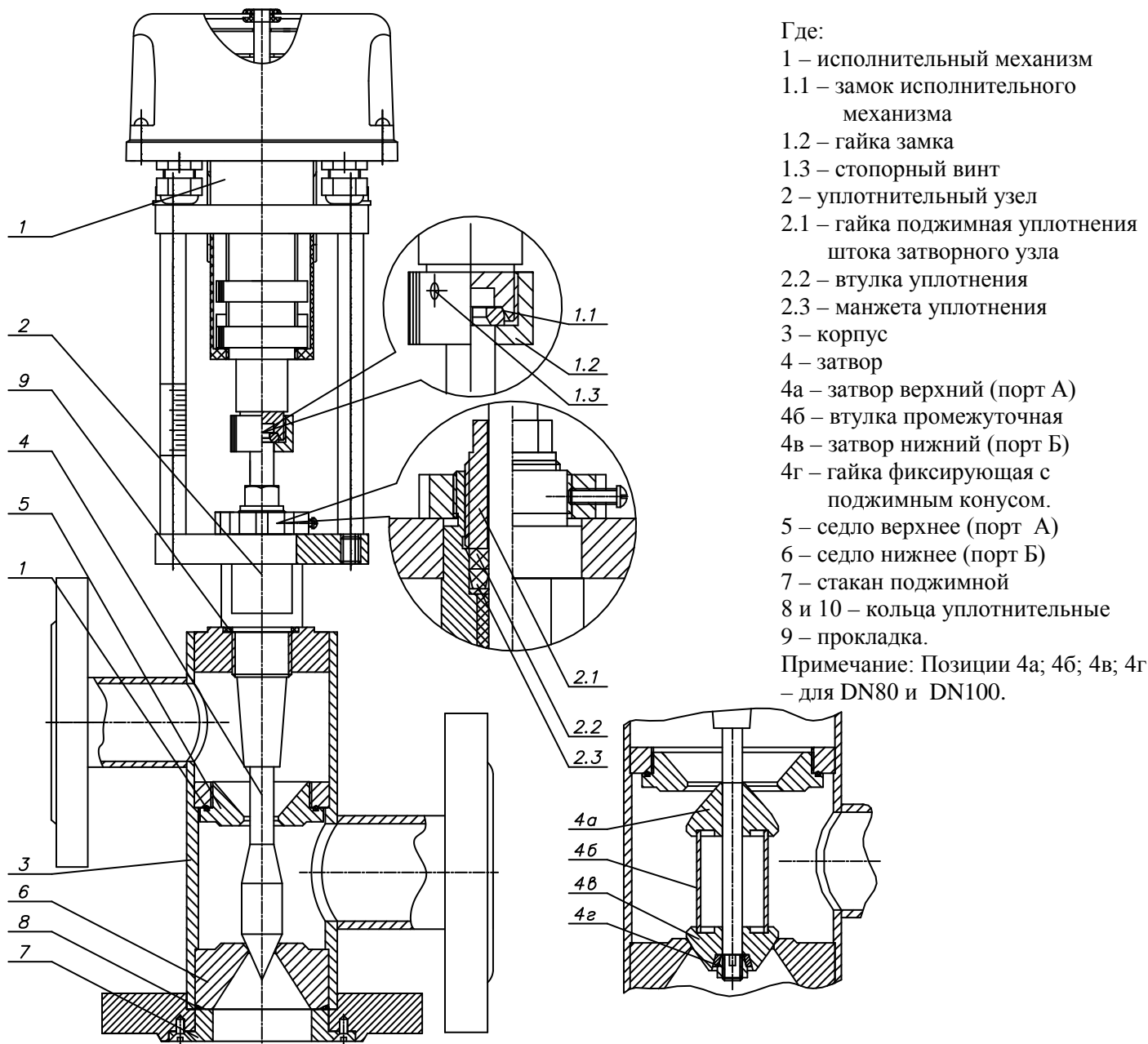
Рисунок 1. Общее устройство клапана смесительного трехходового КСТ-XX(X)/XX.Б-XX
