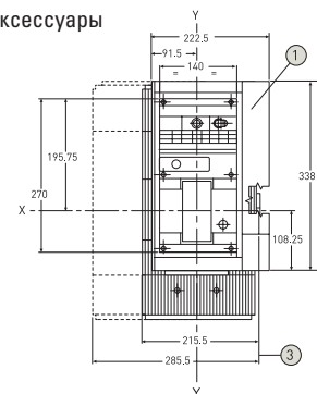
① Передний фланец для двери шкафа (прилагается)
