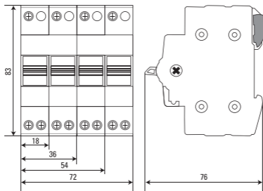
Рис.1 - Габаритные размеры
